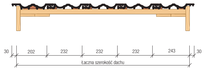
Detal krawędzi dachu z dachówką dwufalową.
