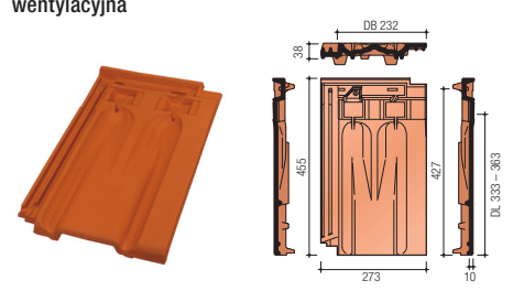
dwufalowa
