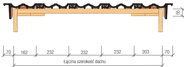
Detal krawędzi dachu z dachówkami szczytowymi.
