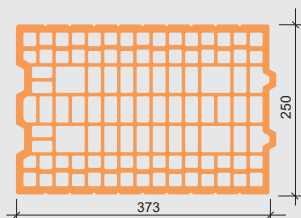
Przekrój pustaka Porotherm 25 Klima+ Profi
