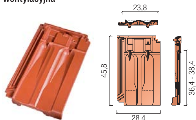
wentylacyjna
